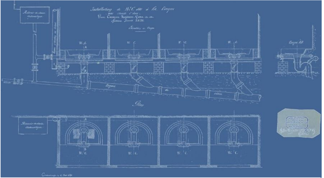
Şekil 6. CH. Dalmas'ın Umumi Alaturka Tuvalet Kurulum Planı
